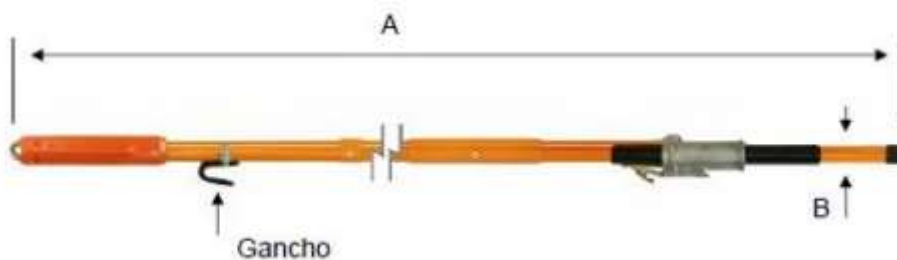
Figura 5: Bastão Pega Tudo
