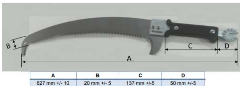
Figura 19: Serra Para Poda Com Adaptador Universal - Dimensões Aproximadas
